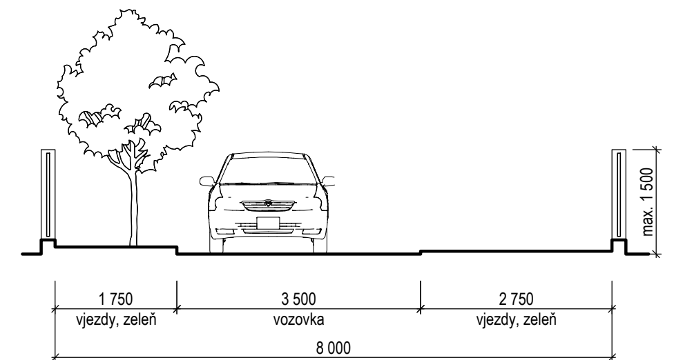
SCHÉMA ZKLIDNĚNÉ KOMUNIKACE 1:75
